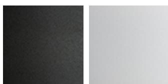
GF69 ? ? ? ? ? GF71 ? ? ? ? ?
